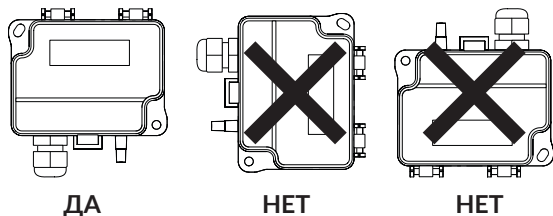
Рисунок 1а - Направление монтажа
