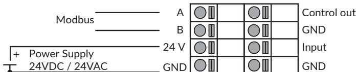
Рисунок 2а - Монтажная электросхема
