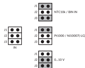
Рисунок 3 - Настройка входного сигнала
