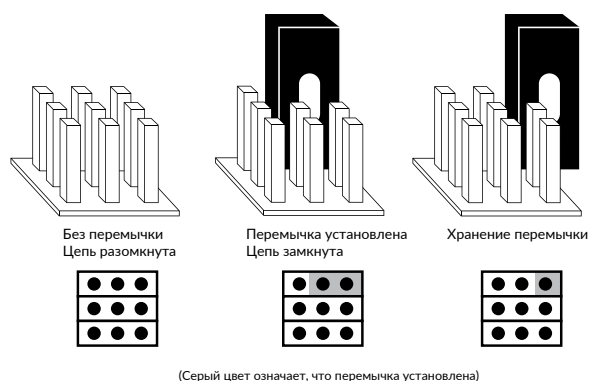
Рисунок 3 - Установка перемычки
