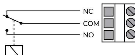
Рисунок 2c - Монтажная электросхема: Реле
